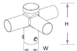
R60-SP3-90-D
